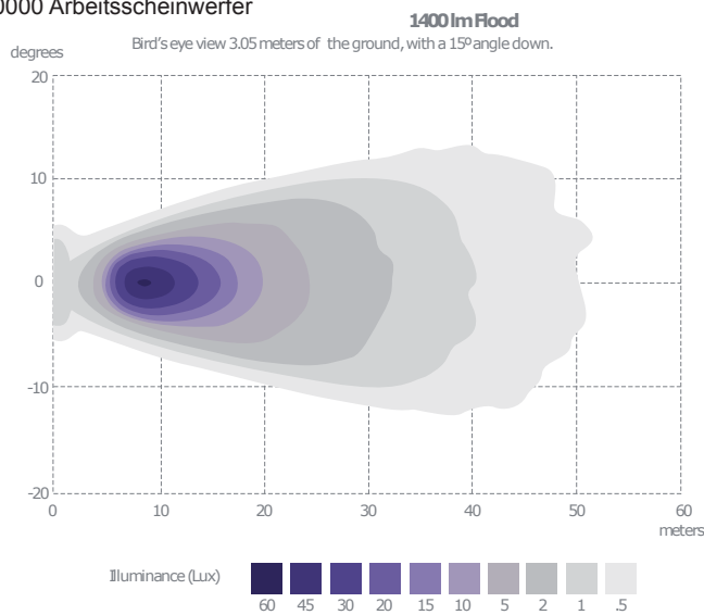
W1500000 Arbeitscheinwerfer
